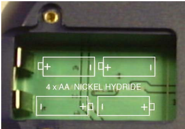
Fig. 2: Vano batterie
